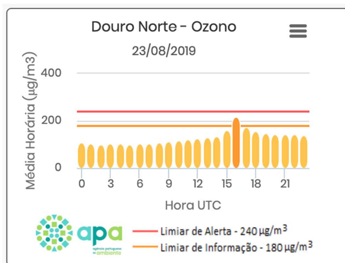
Figura 1. Exemplo da evolução diária das concentrações de O 3 (estação Douro Norte).
