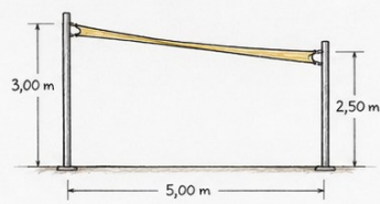
VISTA LATERAL
