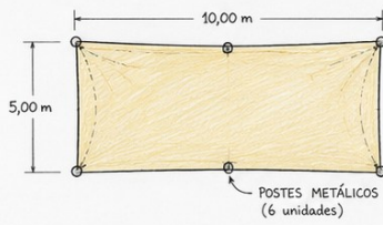
PLANTA (VISTA SUPERIOR)
